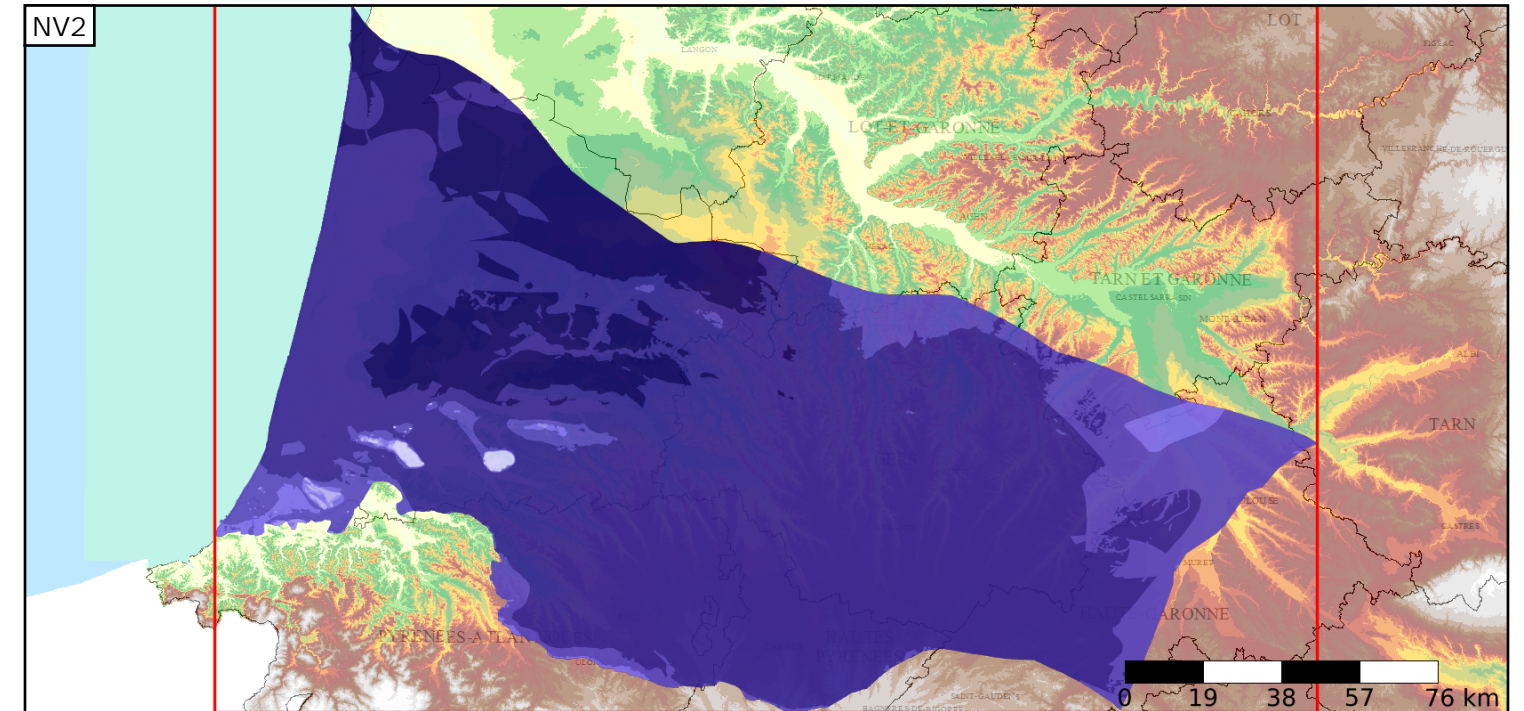
Est incluse dans l'Entité Hydrogéologique 364 Grand domaine hydrogéologique des argiles, évaporites et ophites du Trias du sud du bassin Adour Garonne
